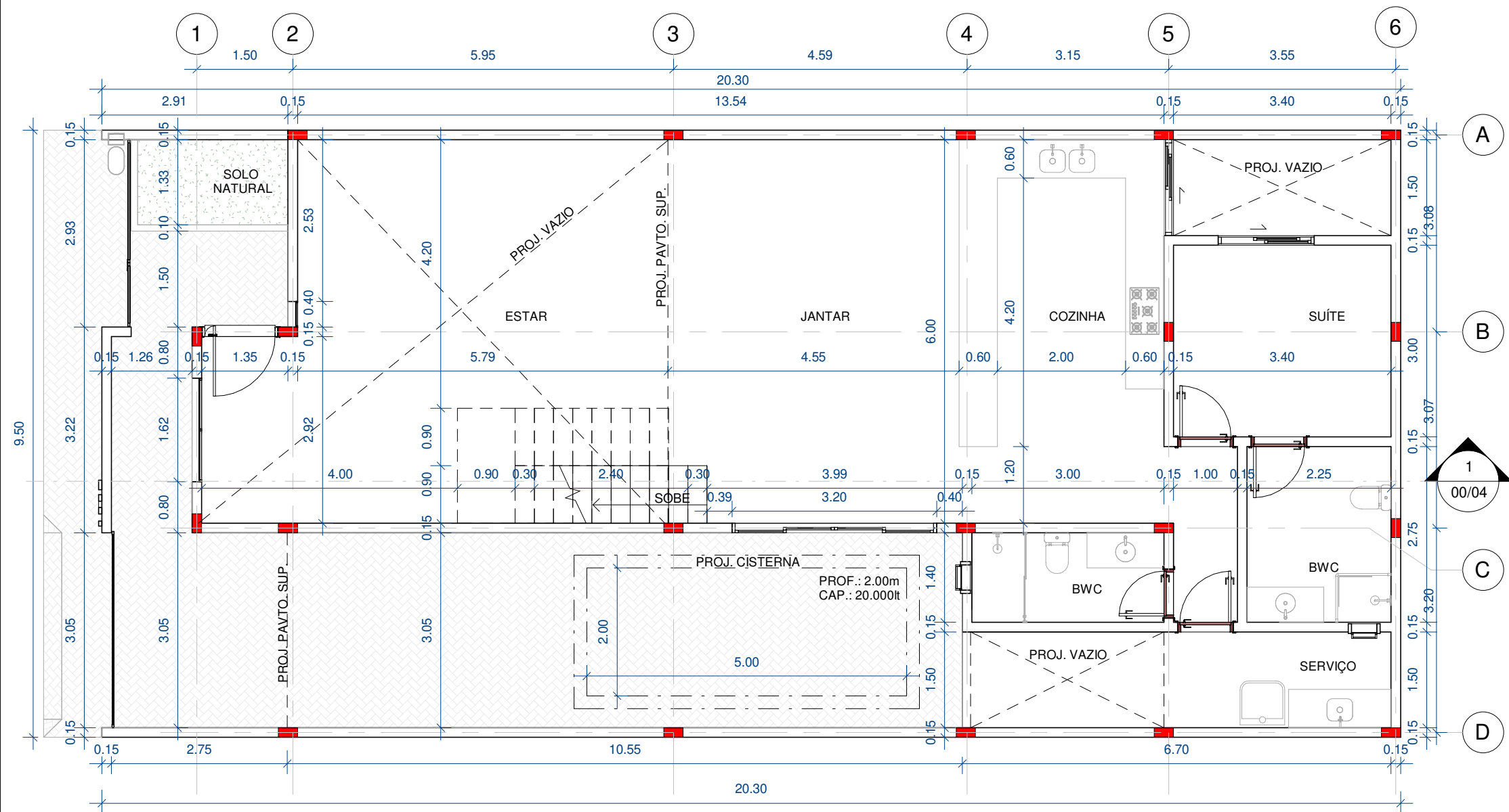
1 PLANTA CONSTRUTIVA-TÉRREO Copiar 1 1 : 80
