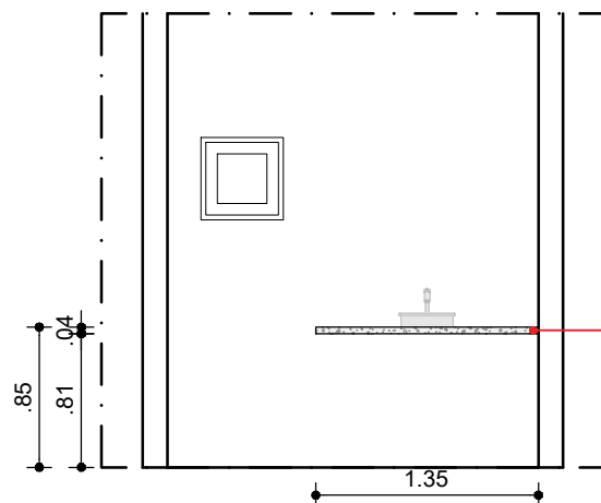
ELEVAÇÃO A - BWC 01
