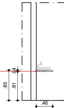
ELEVAÇÃO B - BWC 01
