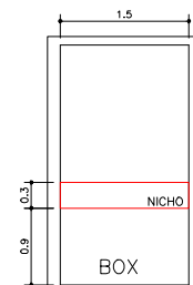
BANHEIRO 05 LARGURA DO BOX ALTURA 0,30M PROF. 0,10M
