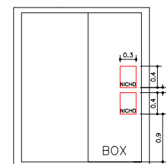
BANHEIRO 06 LARGURA 0,30M ALTURA 0,40M PROF. 0,10M
