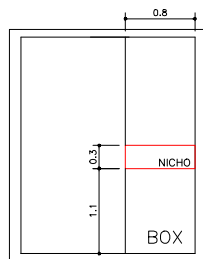
BANHEIRO 01 LARGURA DO BOX ALTURA 0,30M PROF. 0,10M
