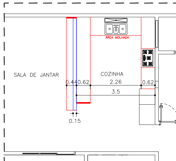
DET. COZINHA – BANCADAS E MURETA MEDIDAS HORIZONTAIS
