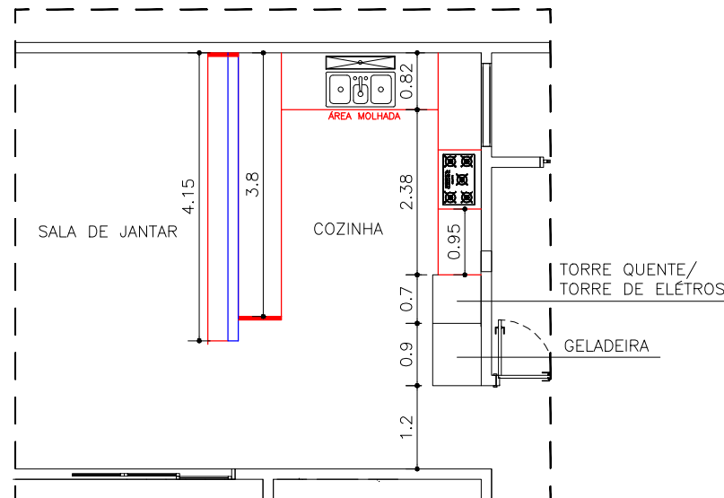
DET. COZINHA – BANCADAS E MURETA MEDIDAS VERTICAIS
