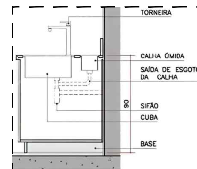
DET. BANCADA – CORTE
