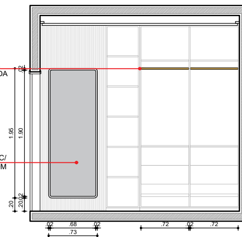
ELEVAÇÃO B - SUÍTE 01
