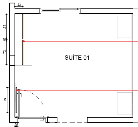
PLANTA BAIXA - SUÍTE 01
