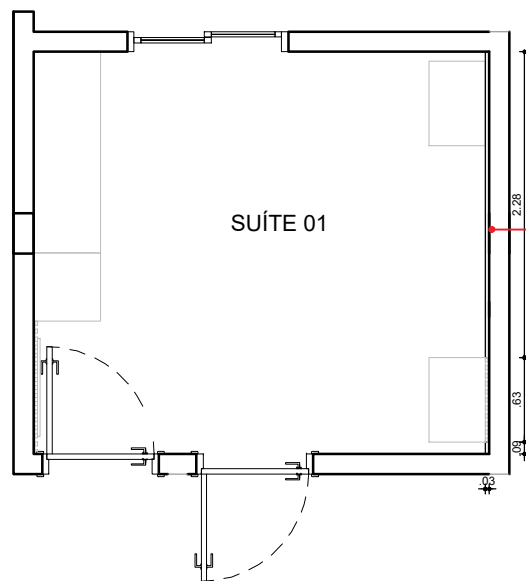
PLANTA BAIXA - SUÍTE 01 ESTOFADOS ESCALA 1/50
