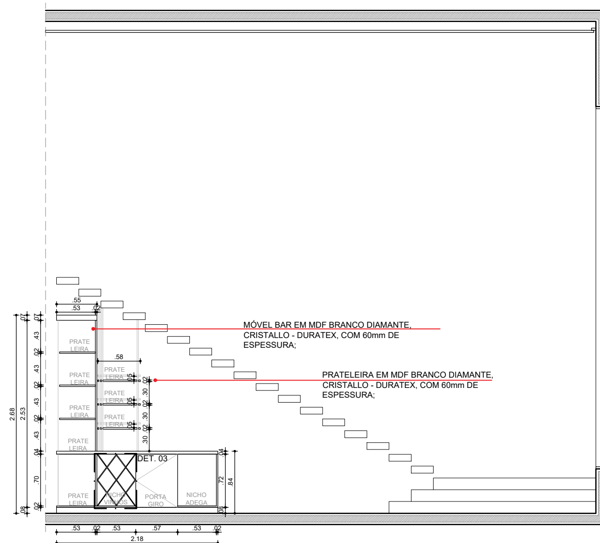
ELEVACÃO C - SALA DE ESTAR E JANTAR MARCENARIA ESCALA 1/50
