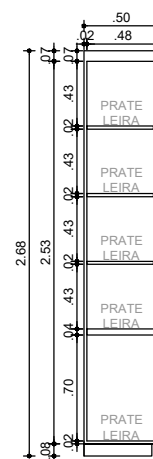
ELEVACÃO C - SALA DE ESTAR E JANTAR MARCENARIA ESCALA 1/50
