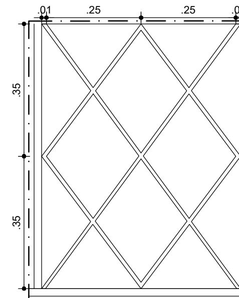
DET. 03 - NICHOS VINHOS MARCENARIA ESCALA 1/5
