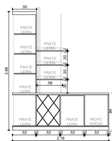
VISTA INTERNA - MÓVEL BAR MARCENARIA ESCALA 1/50
