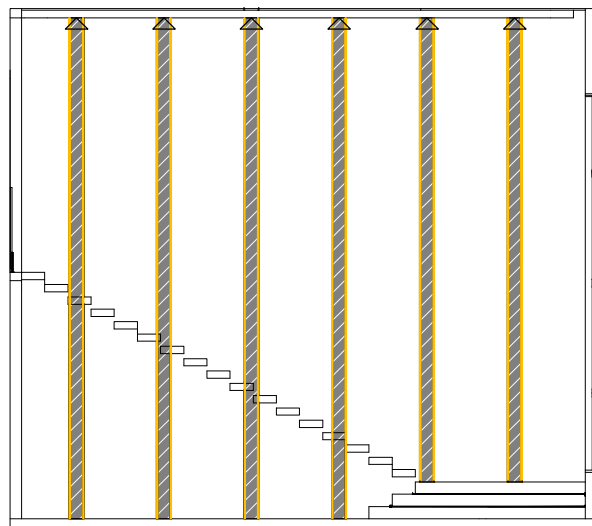
DET. PAREDE ESCADA ESC. 1:100
