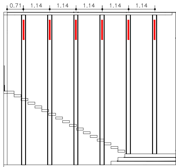
PONTOS ELÉTRICOS - PAREDE ESCADA ESC. 1:100
